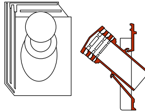
doorvoerpan + ventilatiekoker (met doorvoer voor dakhelling 25° – 45°)
